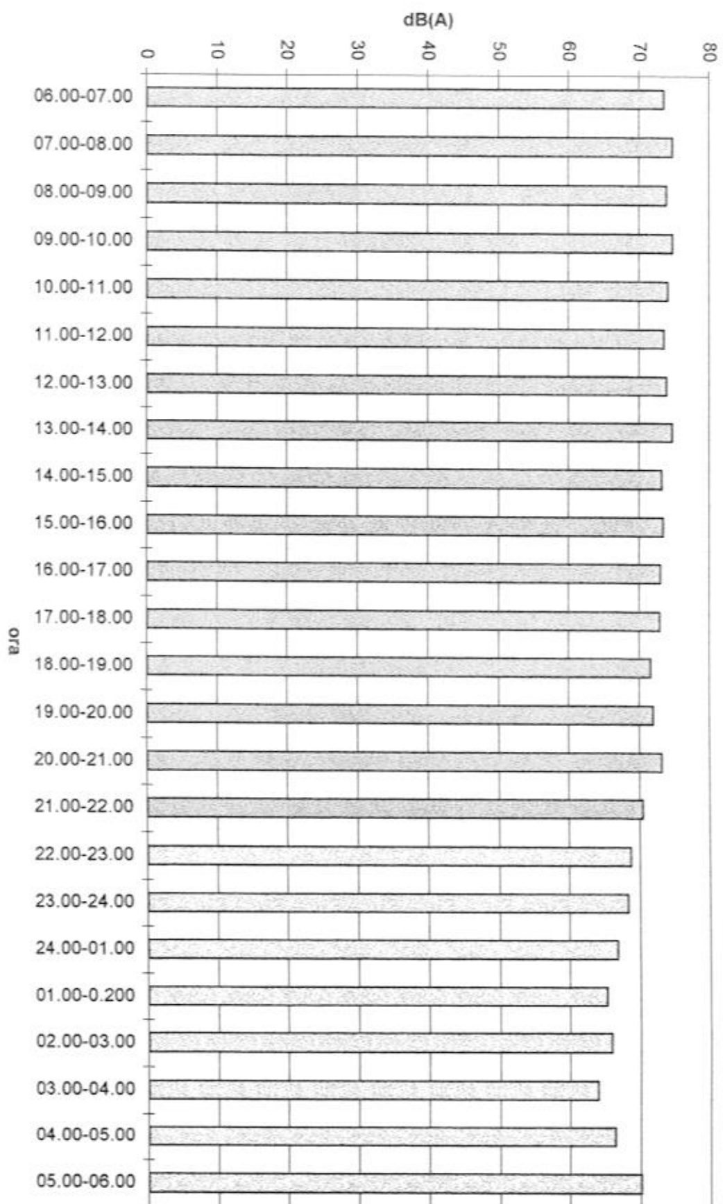
Leq(A) orario diurno e notturno 27/02/2001
